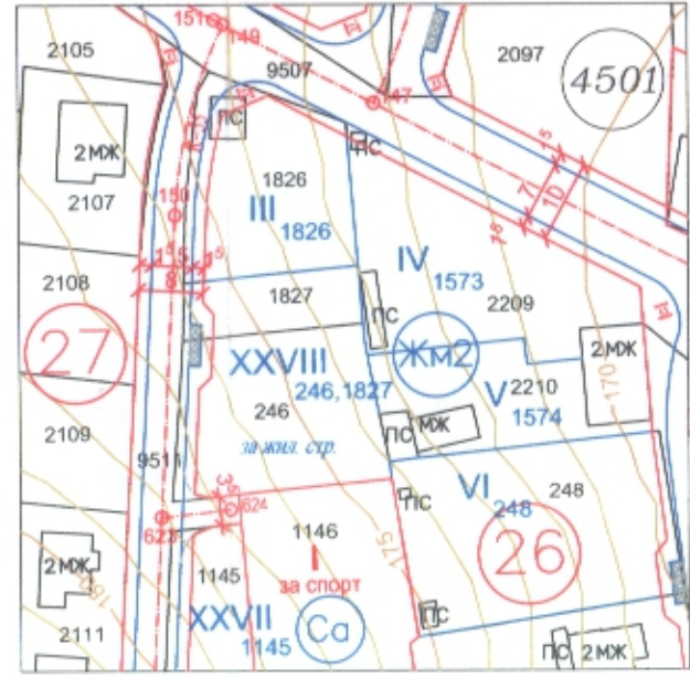
План за регулация М 1:1000
