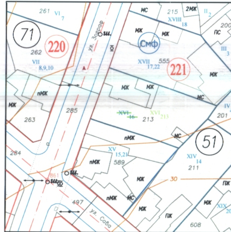
ПЛАН ЗА РЕГУЛАЦИЯ М 1:500
