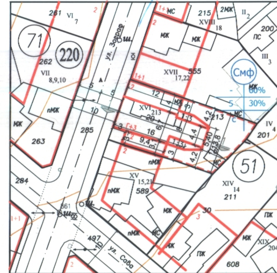
ПЛАН ЗА ЗАСТРОЯВАНЕ М 1:500
