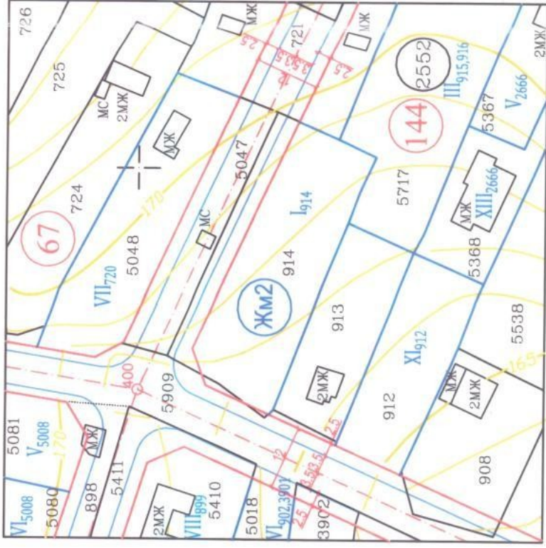
ПОДРОБЕН УСТРОЙСТВЕН ПЛАН /ПУП/- ПЛАН ЗА РЕГУЛАЦИЯ /ПР/
