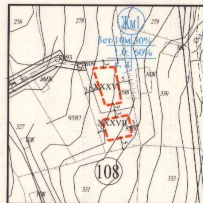
ПЛАН ЗА ЗАСТРОЯВАНЕ НА УПИ XXXVI 9588 и УПИ XXXVII 9588 , КВ. 108 М 1:1000
