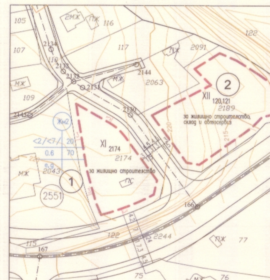
ПЛАН ЗА РЕГУЛАЦИЯ И ЗАСТРОЯВАНЕ
