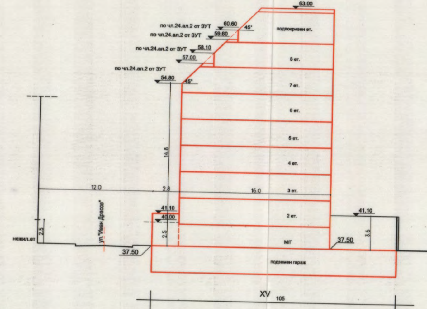
Разрез 2-2 М1:250
