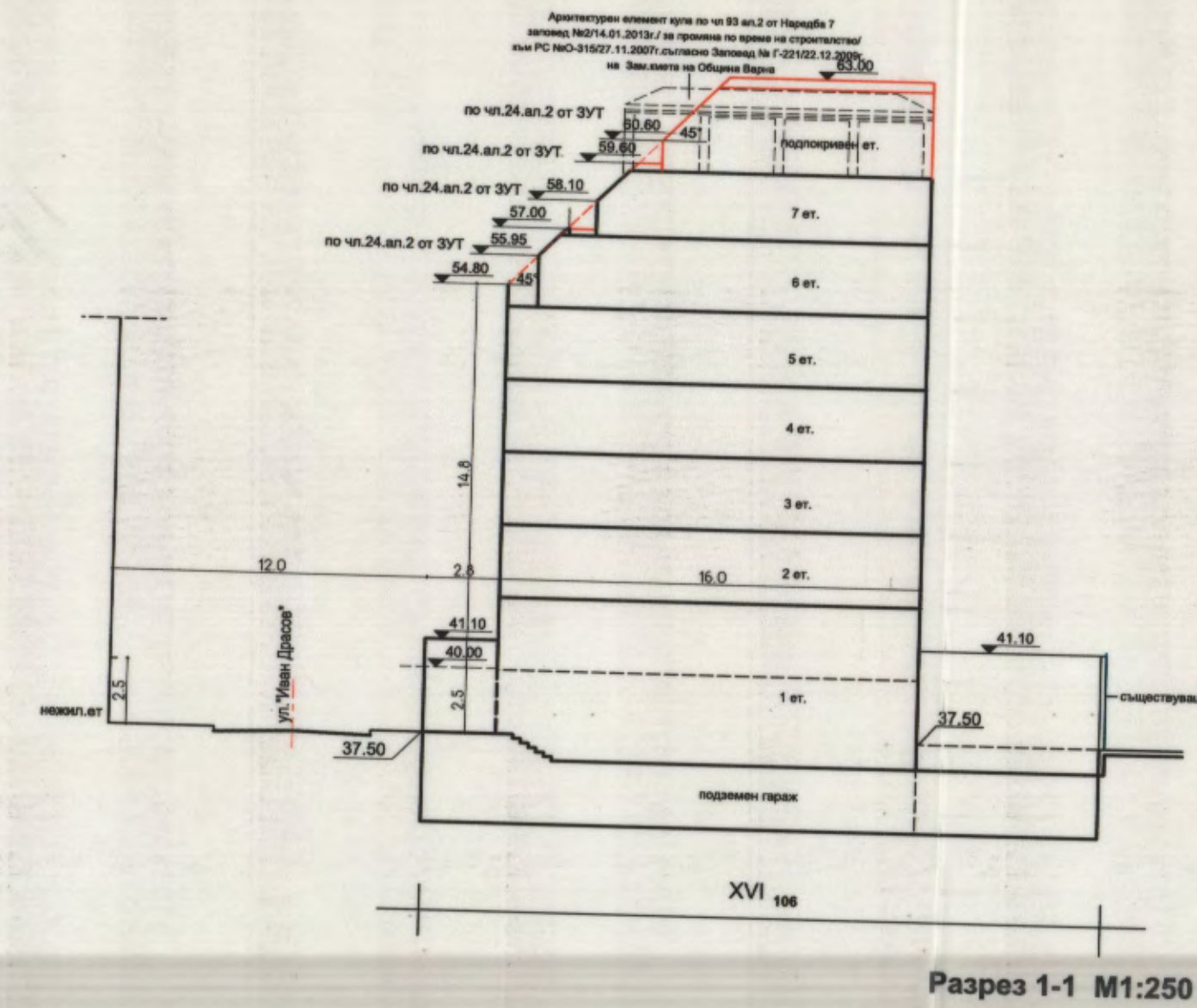
Разрез 1-1 М1:250
