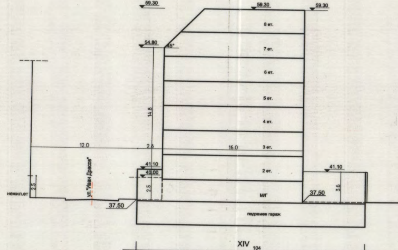
Разрез 3-3 М1:250
