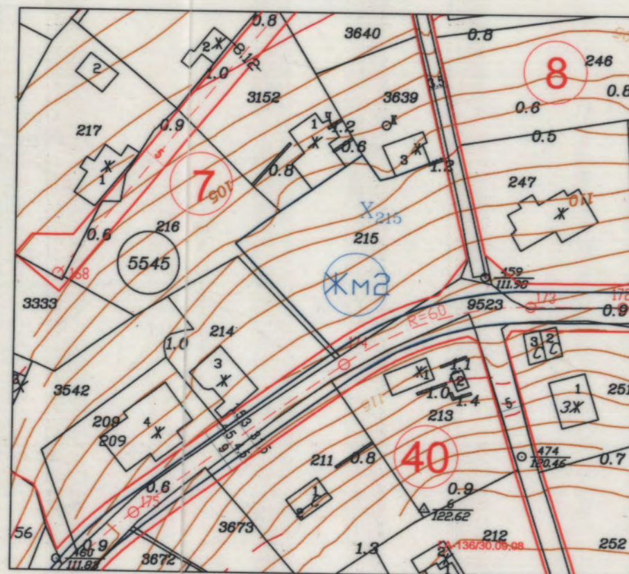
ПЛАН за РЕГУЛАЦИЯ на УПИ Х-215 /ПИ10135.5545.215 по КК/, кв.7 по плана на СО "Зеленика", гр. Варна М 1 : 1000
