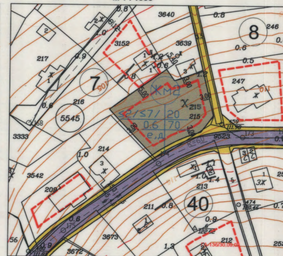
ПЛАН за РЕГУЛАЦИЯ и ЗАСТРОЯВАНЕ на УПИ Х-215 /ПИ10135.5545.215 по КК/, кв.7 по плана на СО "Зеленика", гр. Варна М 1 : 1000
