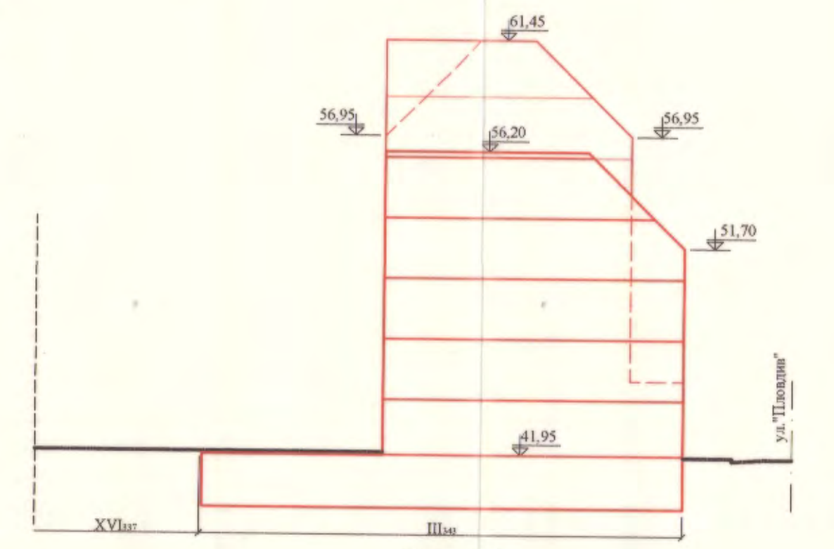
Разрез 1-1 М 1:250
