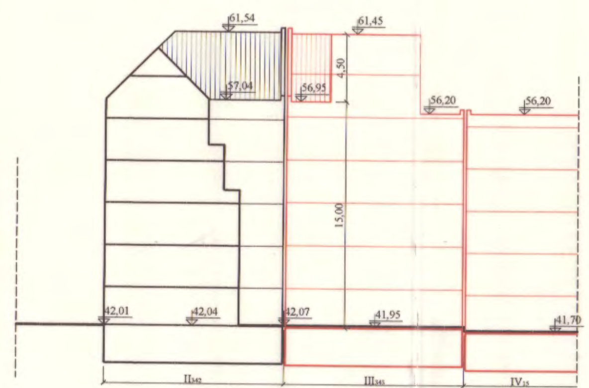
Силует от югозапад М 1:250
