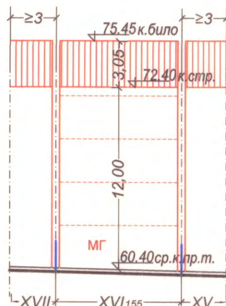
Силует по ул. 'Надежда' М 1:250
