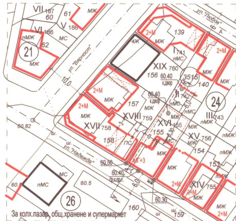
СИТУАЦИЯ М 1:500
