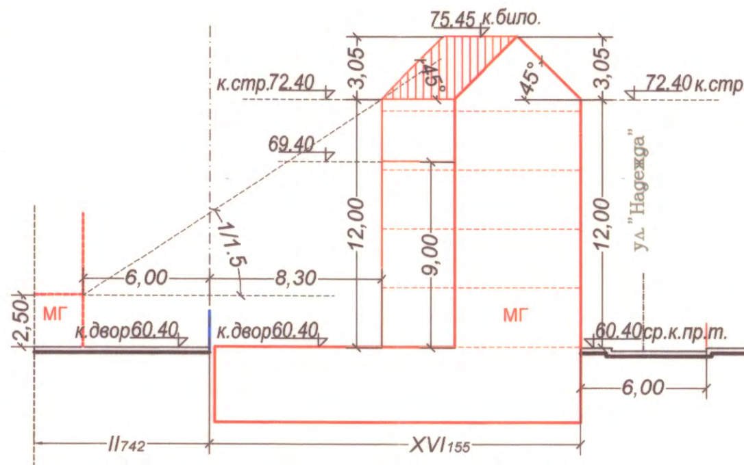
Силует - Разрез А - А М 1:250
