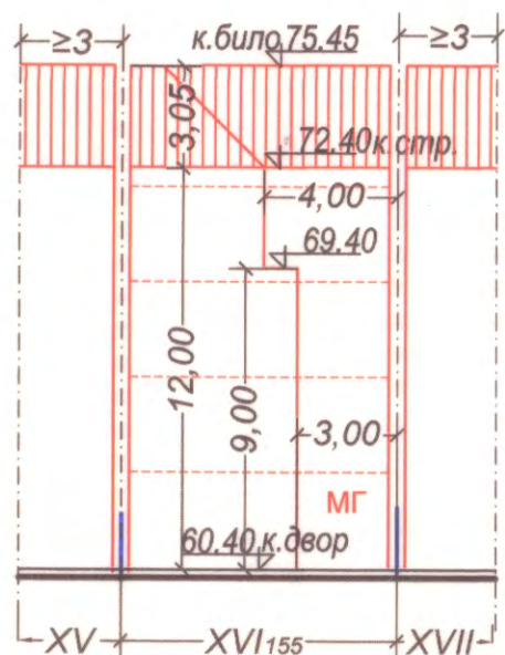
Силует - вътрешен двор М 1:250
